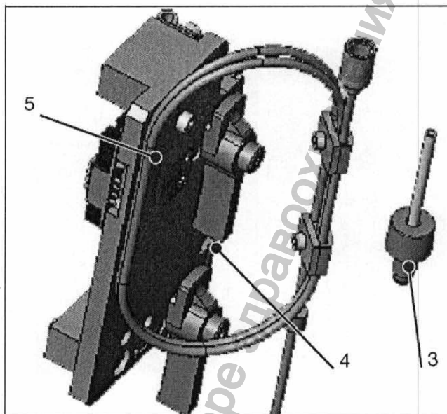
Рис. 9-33: Замена иглы 2
