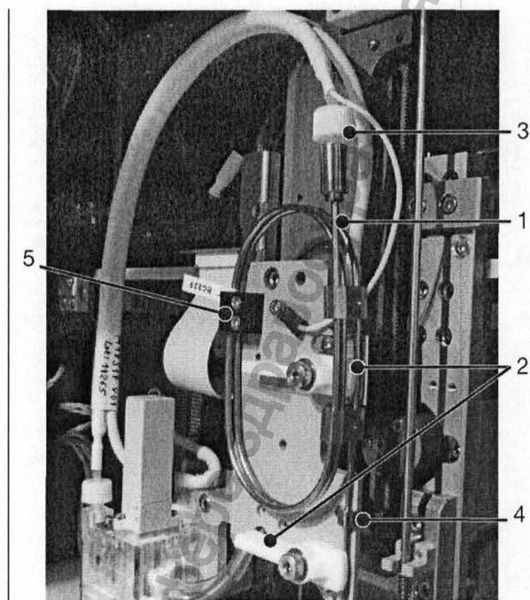
Рис. 9-30: Замена иглы
