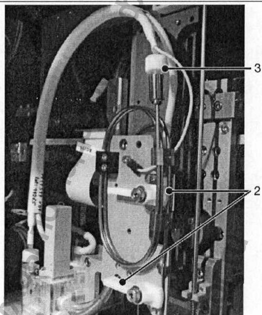
Рис. 9-34: Замена иглы 3
