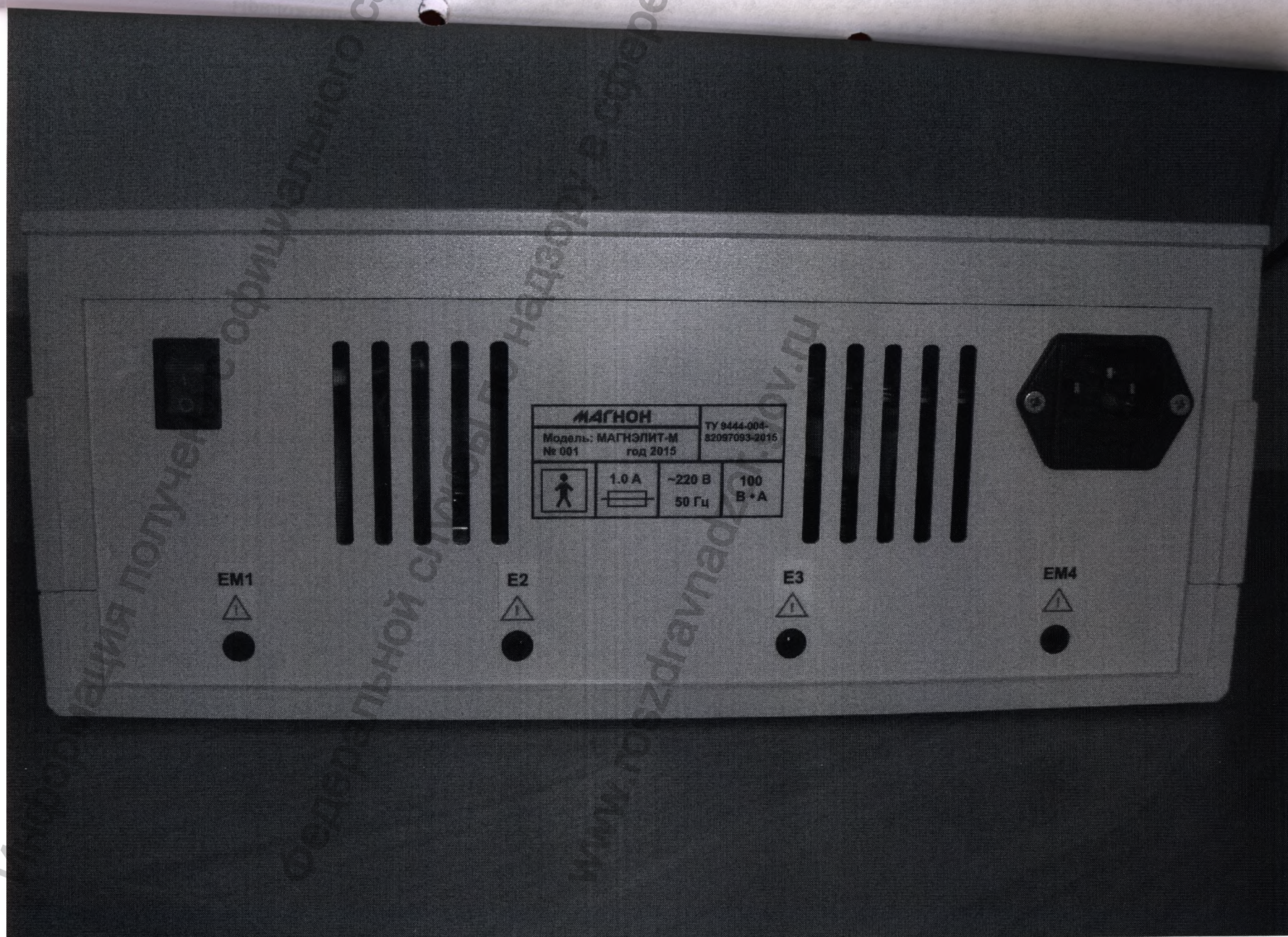
Аппарат электромагнитотерапии "Магнэлит-М" (Задняя панель)
