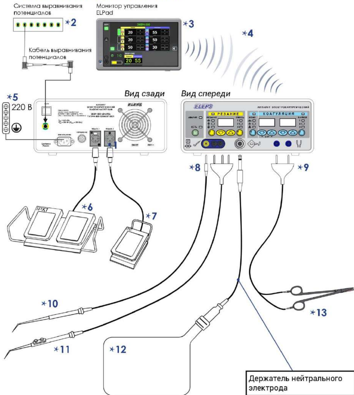
Рисунок 5. Схема подключения принадлежностей к аппарату.
