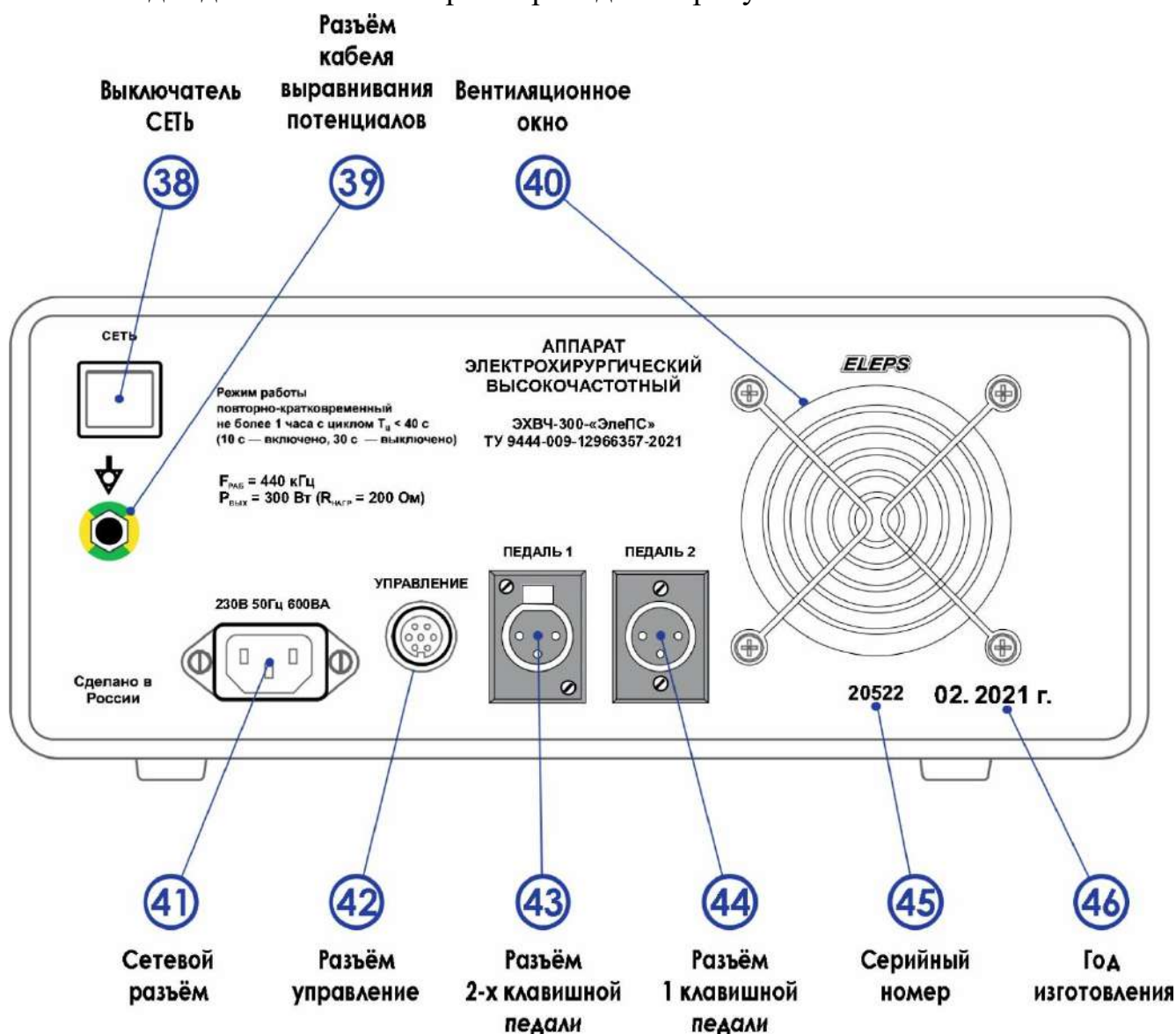
Рисунок 4. Аппарат электрохирургический ЭХВЧ-300-«ЭлеПС». Вид сзади.
