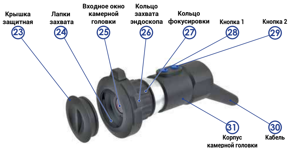
Рисунок 3. Видеокамера эндоскопическая ЭВК-008 4К-«ЭлеПС». Камерная головка исполнение 3.
