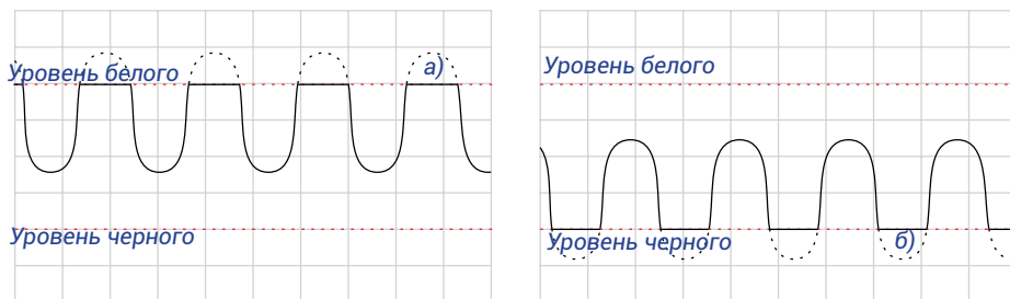
Рисунок 15. Регулировка яркости видеосигнала. а) потеря части информации о светлых участках изображения; б) потеря части информации о темных участках изображения.
