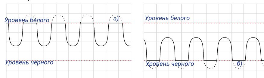
Рисунок 14. Регулировка яркости видеосигнала.
