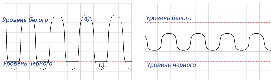
Рисунок 15. Регулировка контрастности видеосигнала. а) потеря части информации о светлых участках изображения; б) потеря части информации о темных участках изображения.
