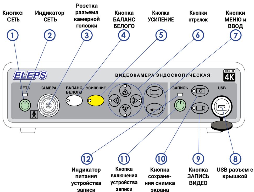
Рисунок 1. Видеокамера эндоскопическая ЭВК-008 4К-«ЭлеПС». Передняя панель блока управления.
