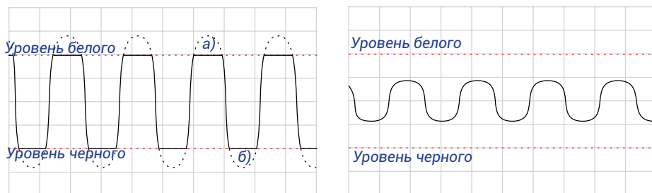
Рисунок 16. Регулировка контрастности видеосигнала. а) потеря части информации о светлых участках изображения; б) потеря части информации о темных участках изображения.
