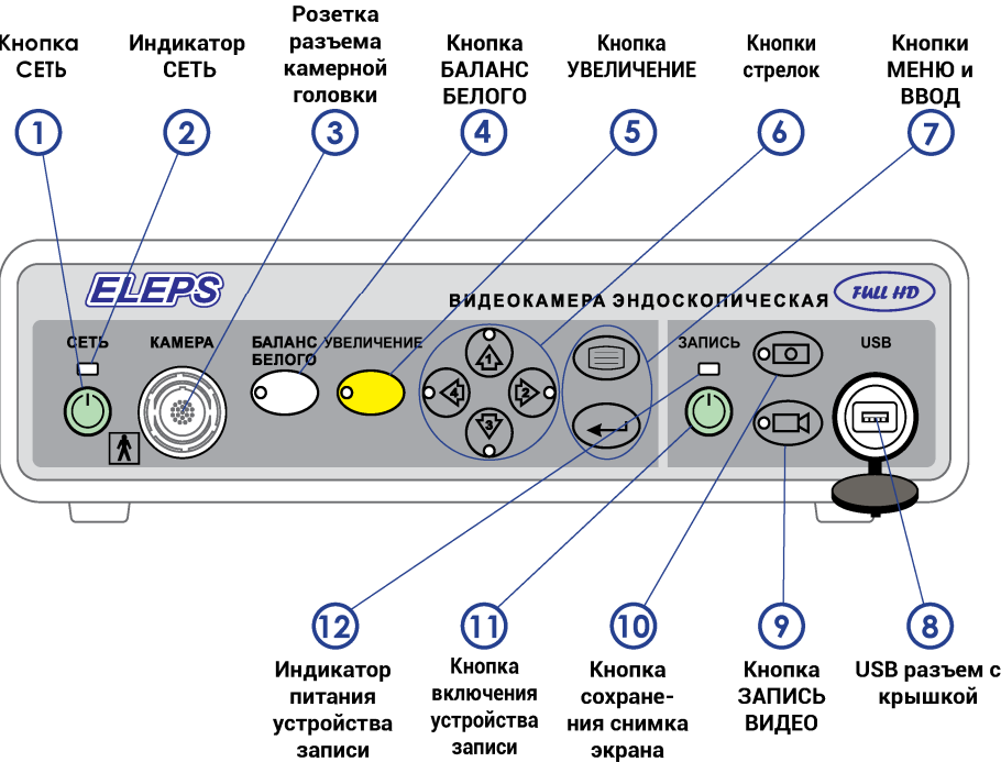
Рисунок 1. Видеокamera эндоскопическая ЭВК-007 Full HD-«ЭлеПС». Передняя панель блока управления.
