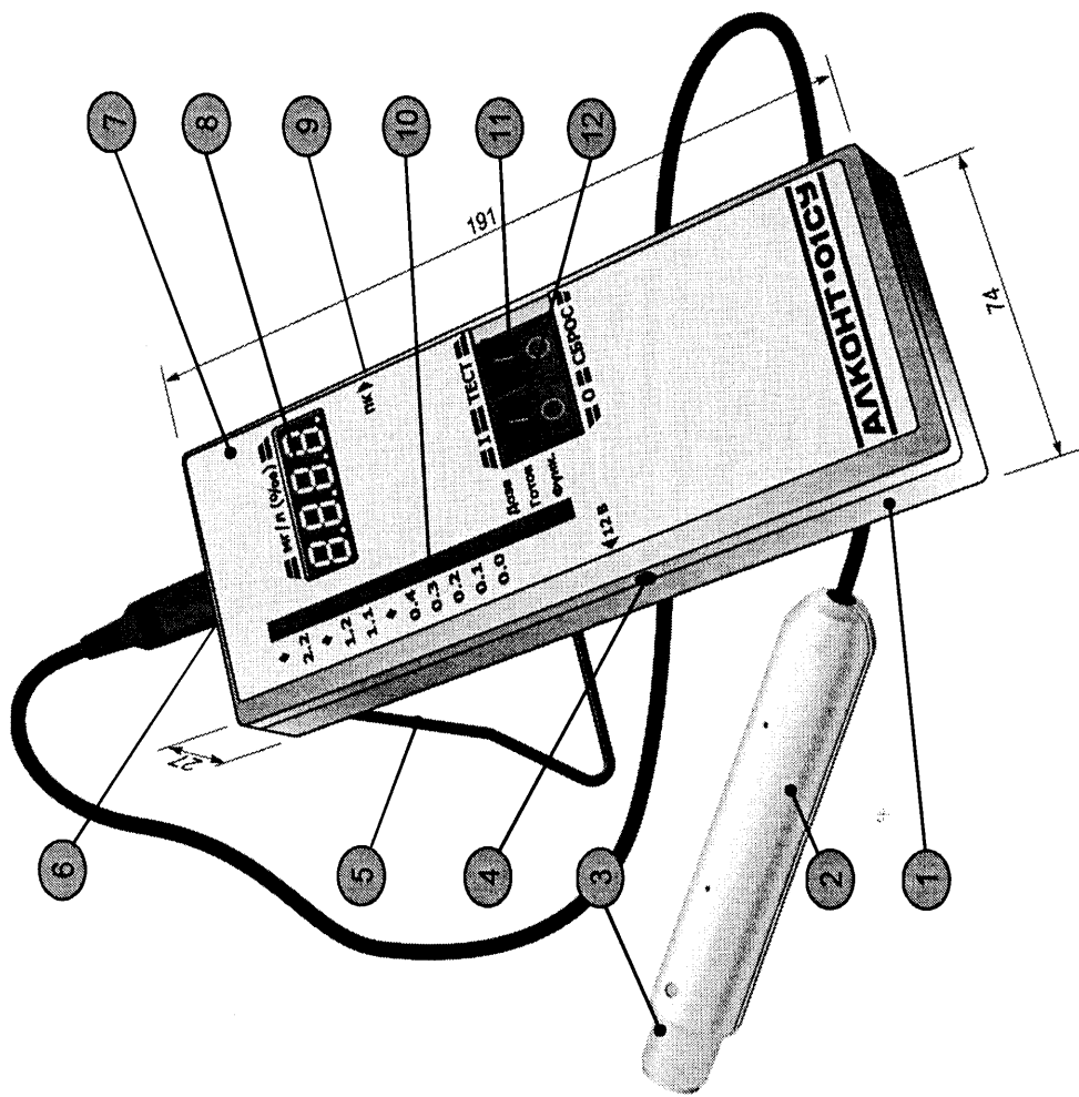
Рис.1. Внешний вид и габаритные размеры прибора «Алkont 01су».
