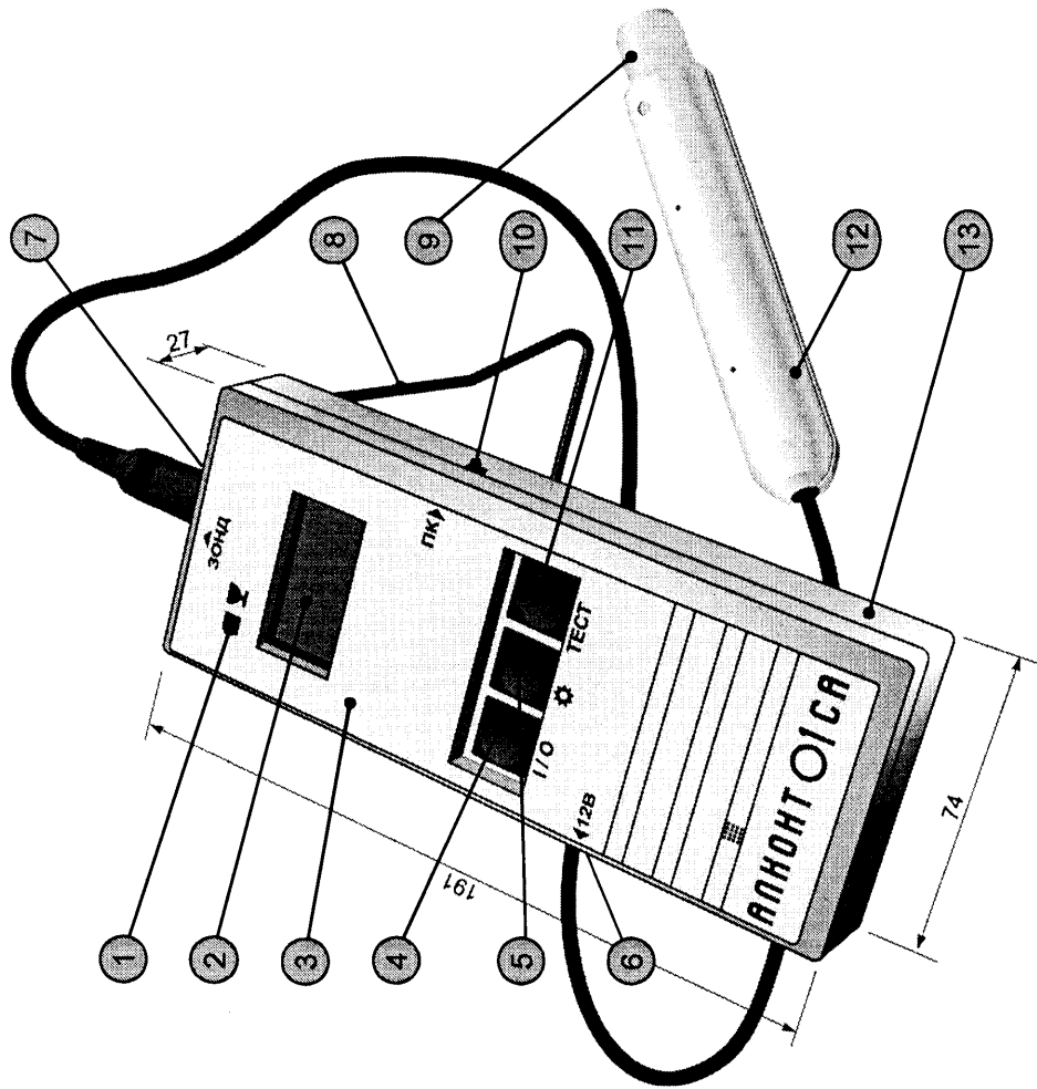
Рис. 1. Внешний вид и габаритные размеры прибора "Алkont 01са".
