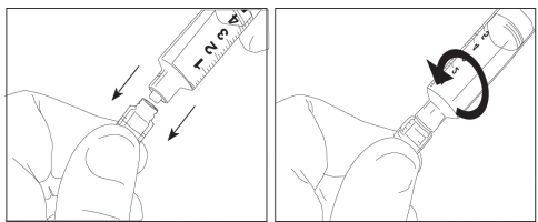
Рис. 3: Винтовой охватываемый коннектор Люэр-Лок (MLL)
