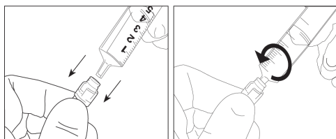
Figur 2: Hann-slipluer (MSL)
