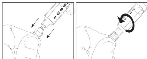
圖 3：旋緊式公接頭 (MLL)
