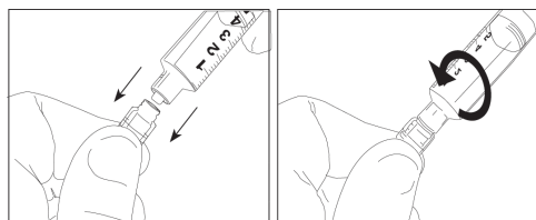
Obr. 3: Koncovka luer typu samec se závitem (MLL)
