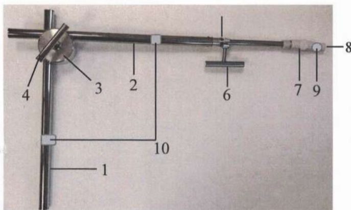
Рисунок 12 Штанга (телескопическая)
