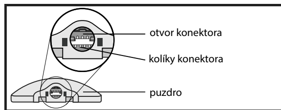
Obrázok 6. Súčasti vysielača
