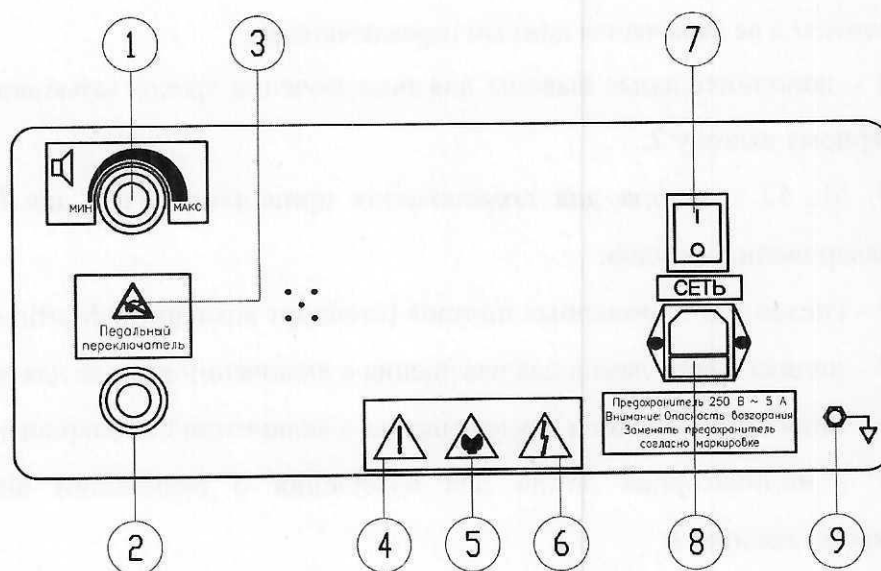
Рисунок 5 – Задняя панель
