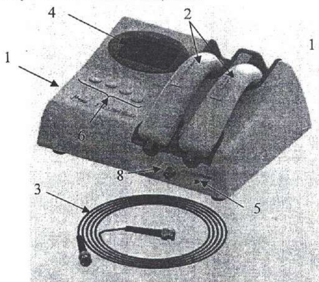
Рисунок 1 Общий вид вариантов исполнения:
