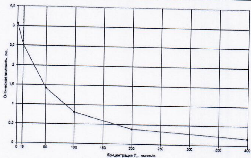
Рис. Пример зависимости оптической плотности от концентрации T_4 общ. в калибровочных образцах.
