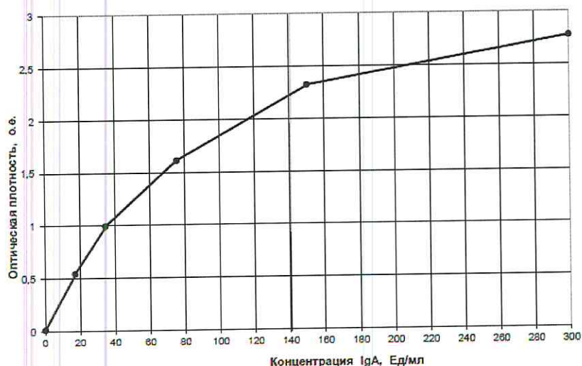
Рис. Зависимость оптической плотности от концентрации IgA общ в калибровочных образцах.
