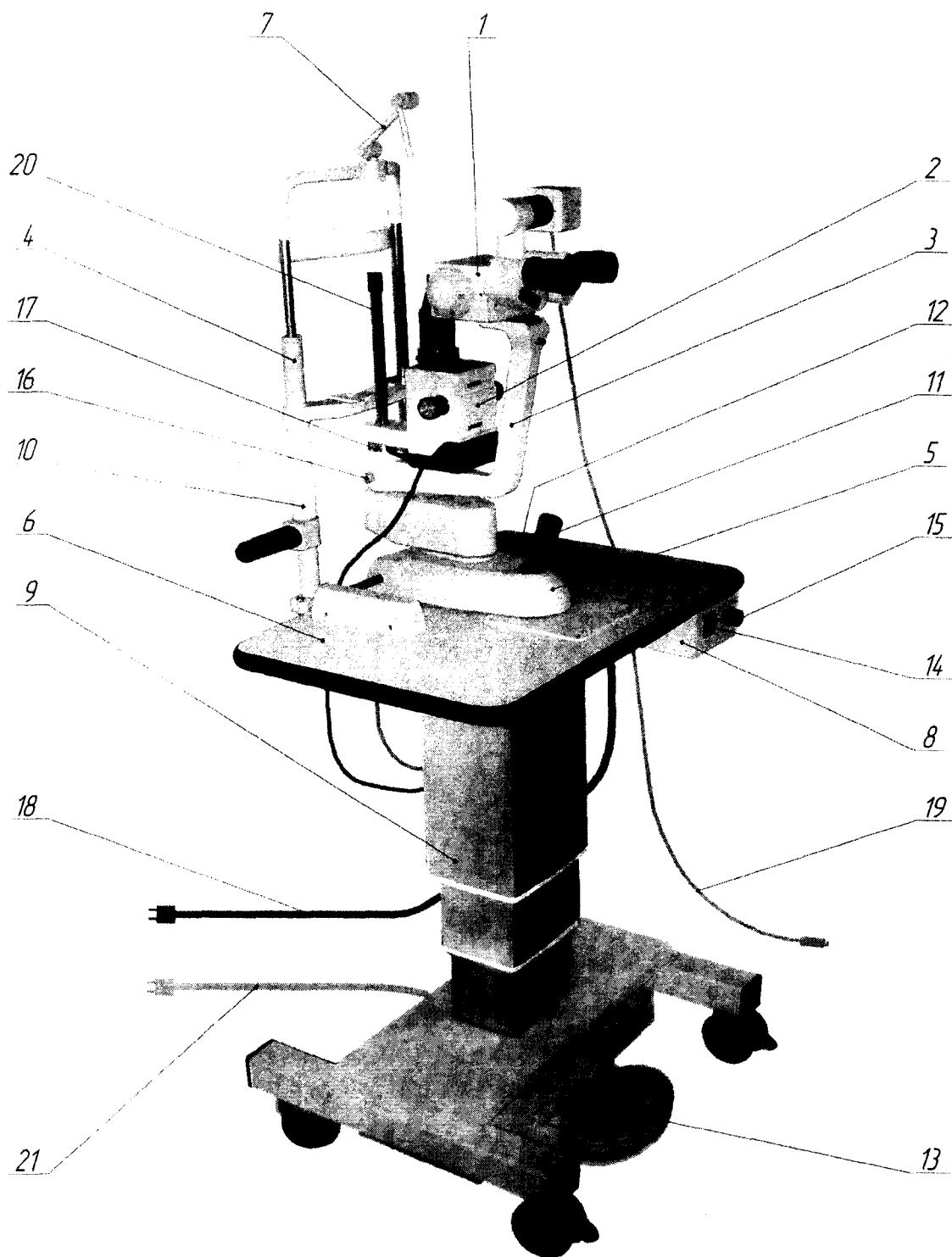
Рисунок 1 - Щелевая лампа ЛС-01-«Зенит»
