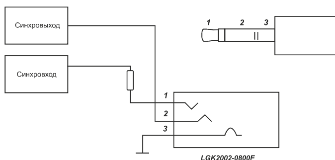
Рис. 24. Распайка разъема
