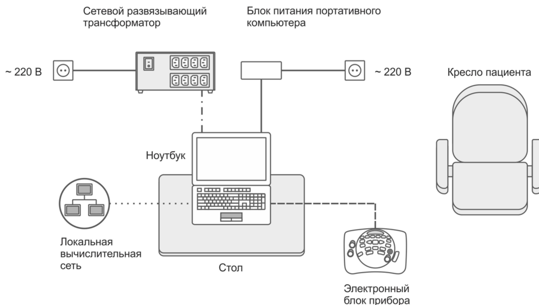
Рис. 11. Примерный план размещения комплекса при подключении к портативному компьютеру (пояснения ниже)
