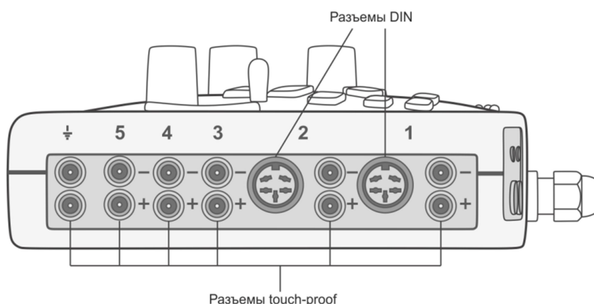
Рис. 2. Внешний вид правой торцевой панели электронного блока
