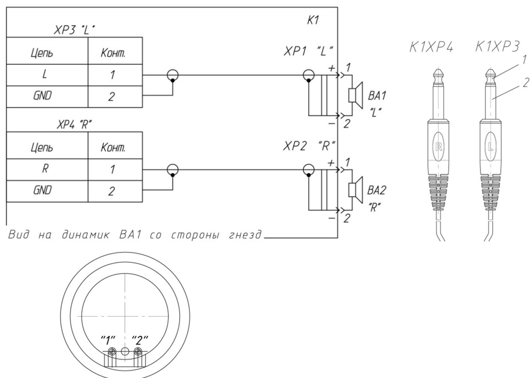
Рис. 21. Схема электрическая принципиальная аудиометрических наушников
