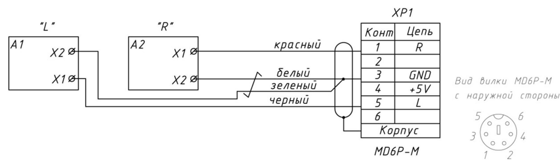
Рис. 22. Схема электрическая принципиальная светодиодных очков
