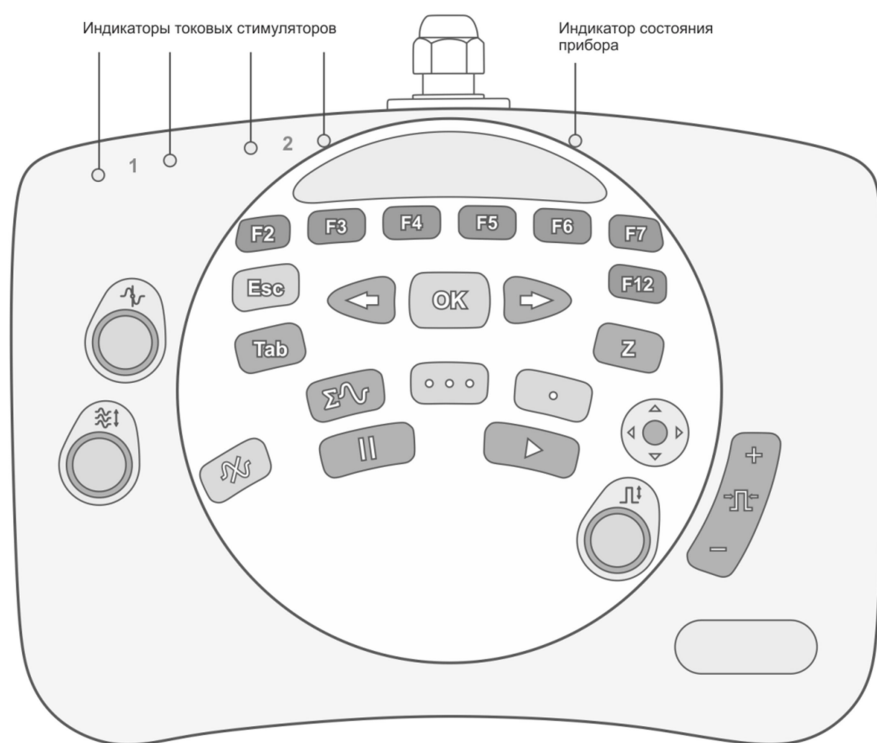
Рис. 6. Функциональная клавиатура электронного блока
