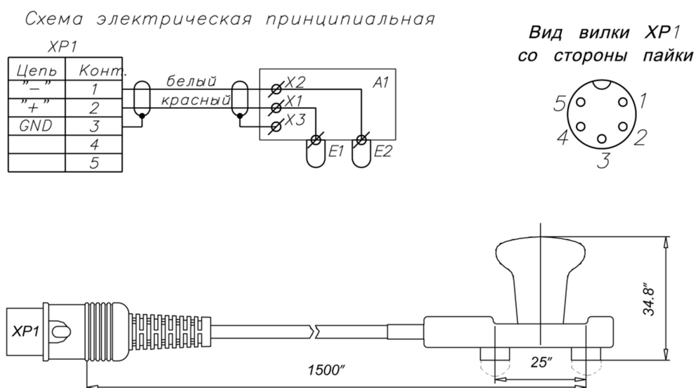
Рис. 23. Схема электрическая принципиальная токового стимулирующего электрода
