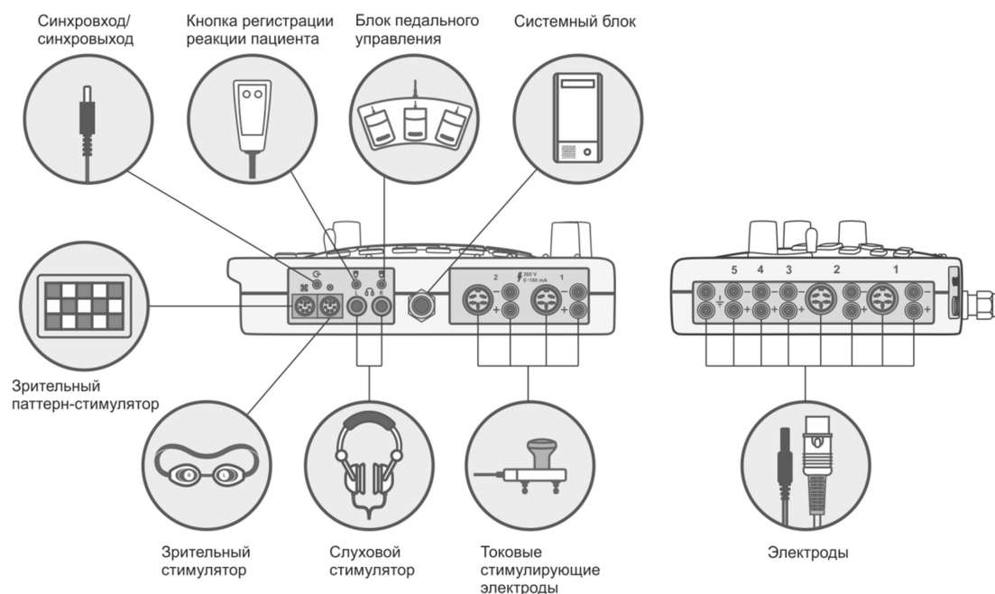
Рис. 12. Подключение электронного блока комплекса к компьютеру
