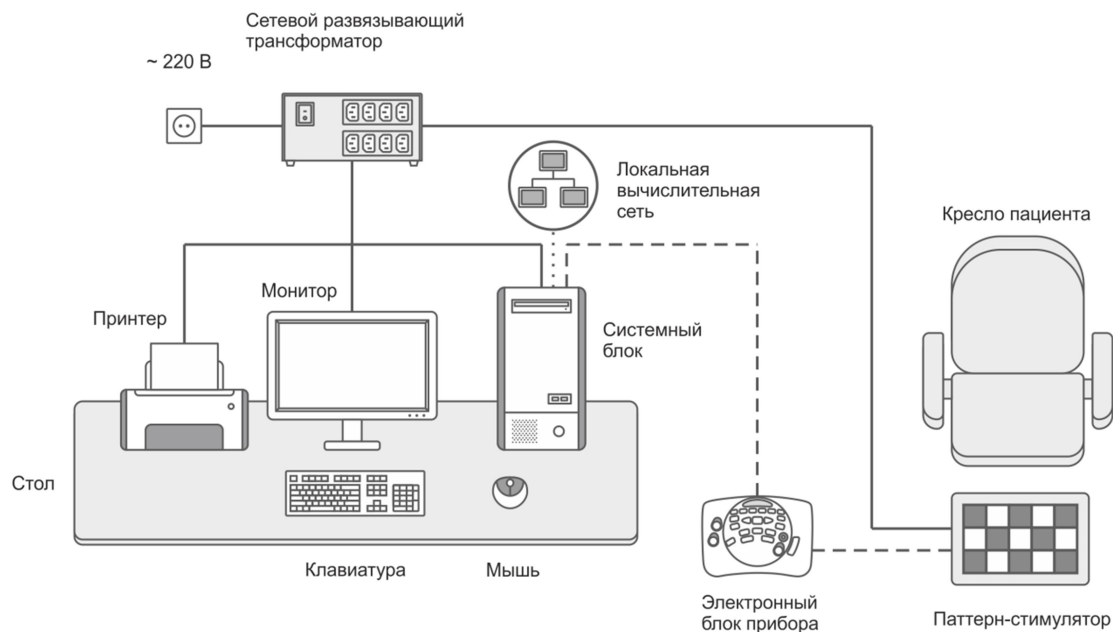
Рис. 10. Примерный план размещения комплекса при подключении к стационарному компьютеру (пояснения ниже)
