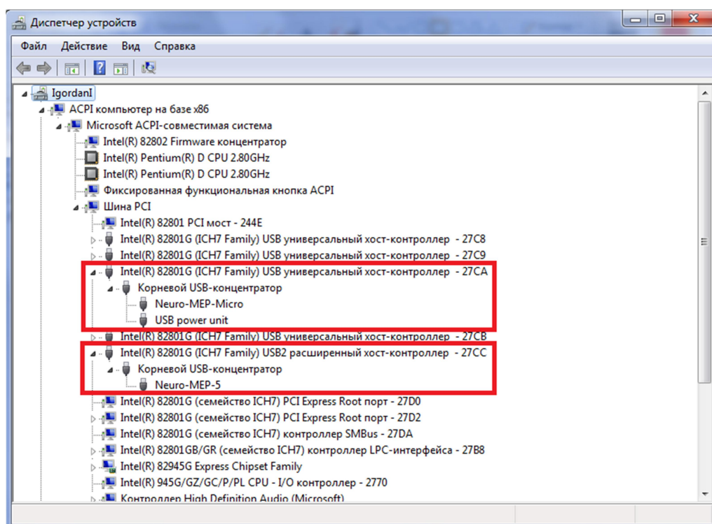
Рис. 20. Неработоспособная конфигурация USB-устройств
