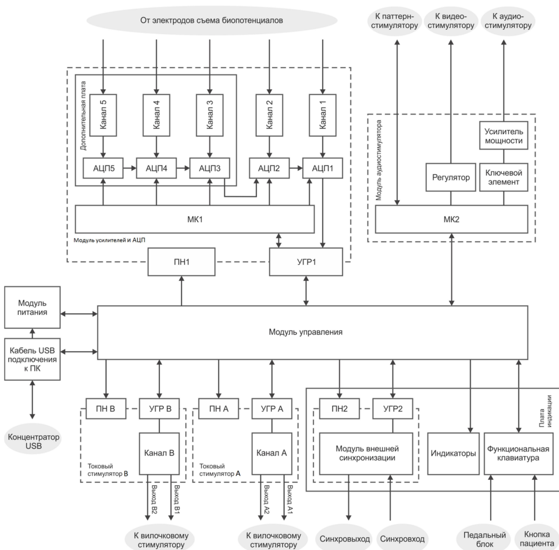
Рис. 1. Структурная схема электронного блока комплекса
