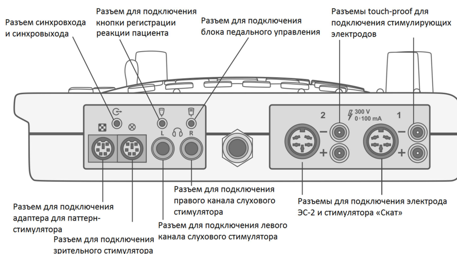
Рис. 3. Внешний вид верхней торцевой панели электронного блока
