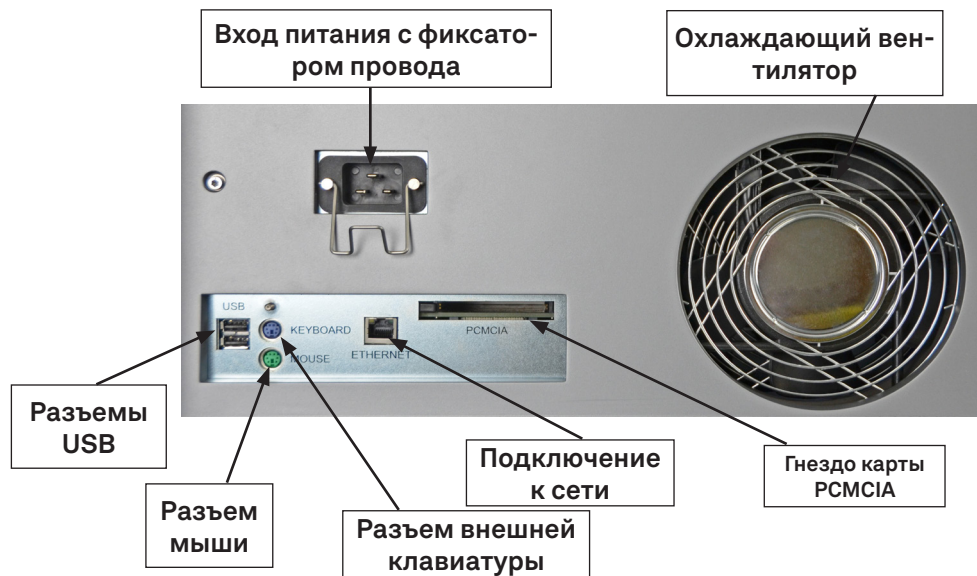
Рисунок 6. Задняя панель.
