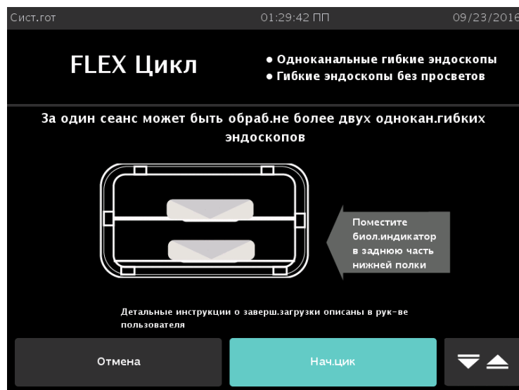
Рисунок 16б. Загрузите камеру для цикла FLEX.
