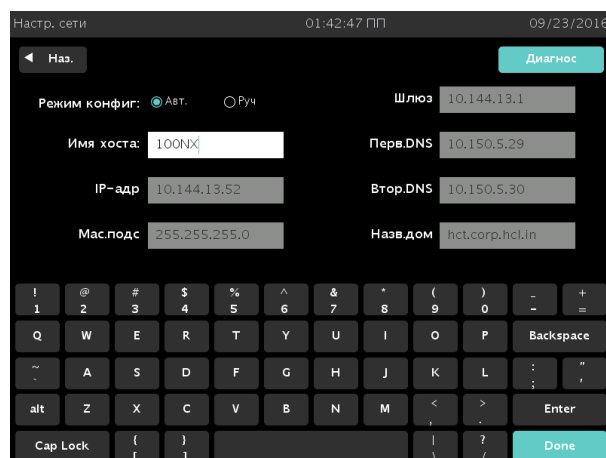
Рисунок 75. Настройки сети 1. Данные в поле этого экрана представлены для контекста.
