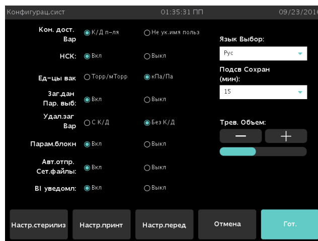
Рисунок 70. Экран «Конфигурация системы».
