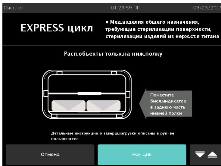
Рисунок 16d. Загрузите камеру для цикла EXPRESS.
