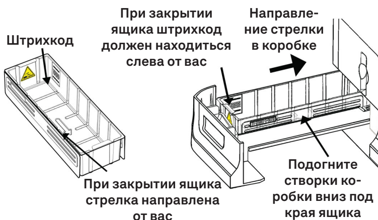
Рисунок 58. Правильное положение коробки для кассет в ящике. Обратите внимание на направление стрелки в коробке.
