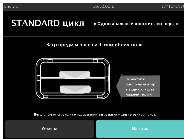
Рисунок 22а. Загрузите камеру для цикла STANDARD.
