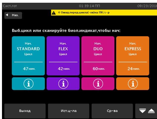
Рисунок 72. Экран «Система готова» показывает циклы для передачи.
