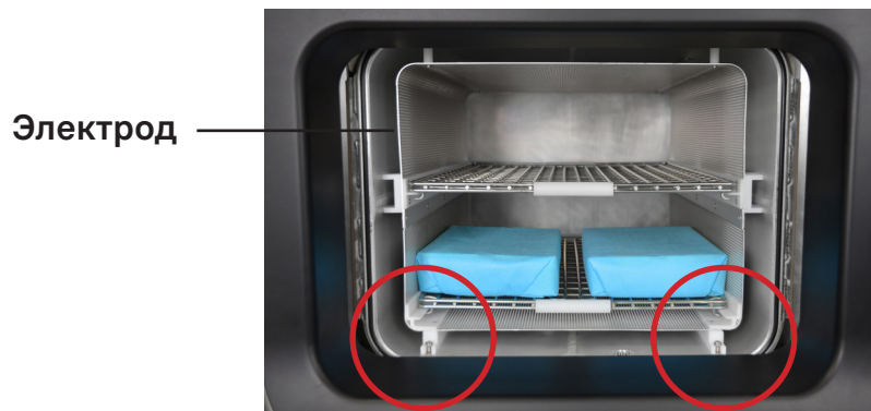
Рисунок 8. Стерилизуемые объекты НЕ должны касаться электрода.
