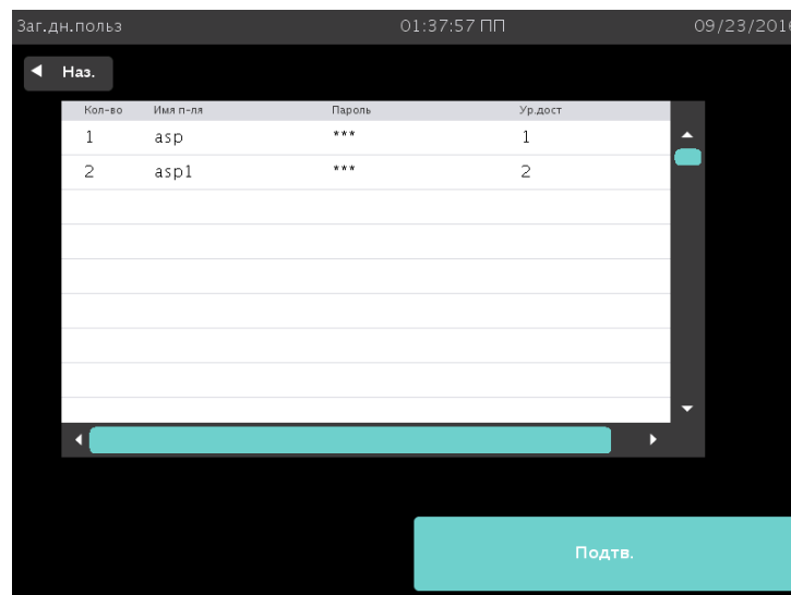
Рисунок 55. Загрузить данные пользователя.
