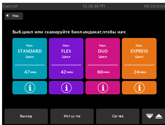
Рисунок 66. Выбор цикла. В вашей системе могут быть другие варианты циклов.
