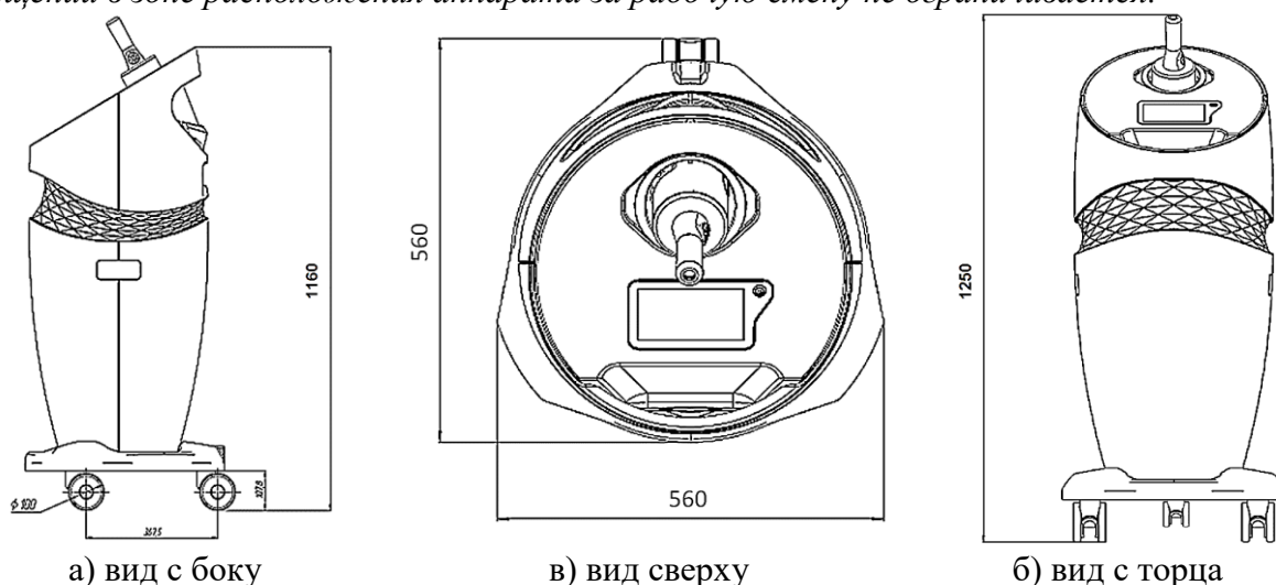
Рисунок 5 – Габаритные размеры устройства в вариантах исполнения IV и V
