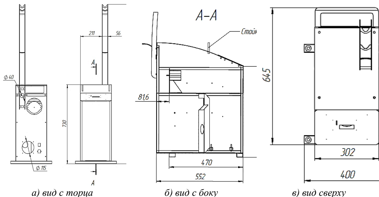
Рисунок 3 – Линейные размеры основного блока в металлическом корпусе
