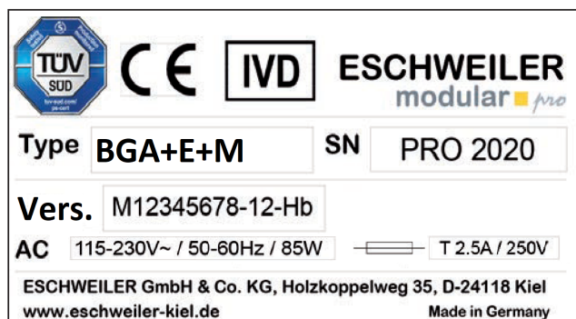
Рисунок 13 Табличка с типом прибора
