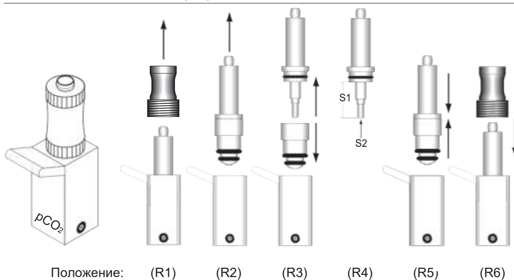
Сенсор p\text{CO}_2 в разобранном виде
