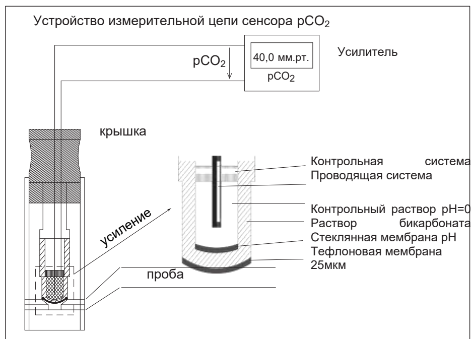
Рисунок 30 Устройство измерительной цепи сенсора p\text{CO}_2
