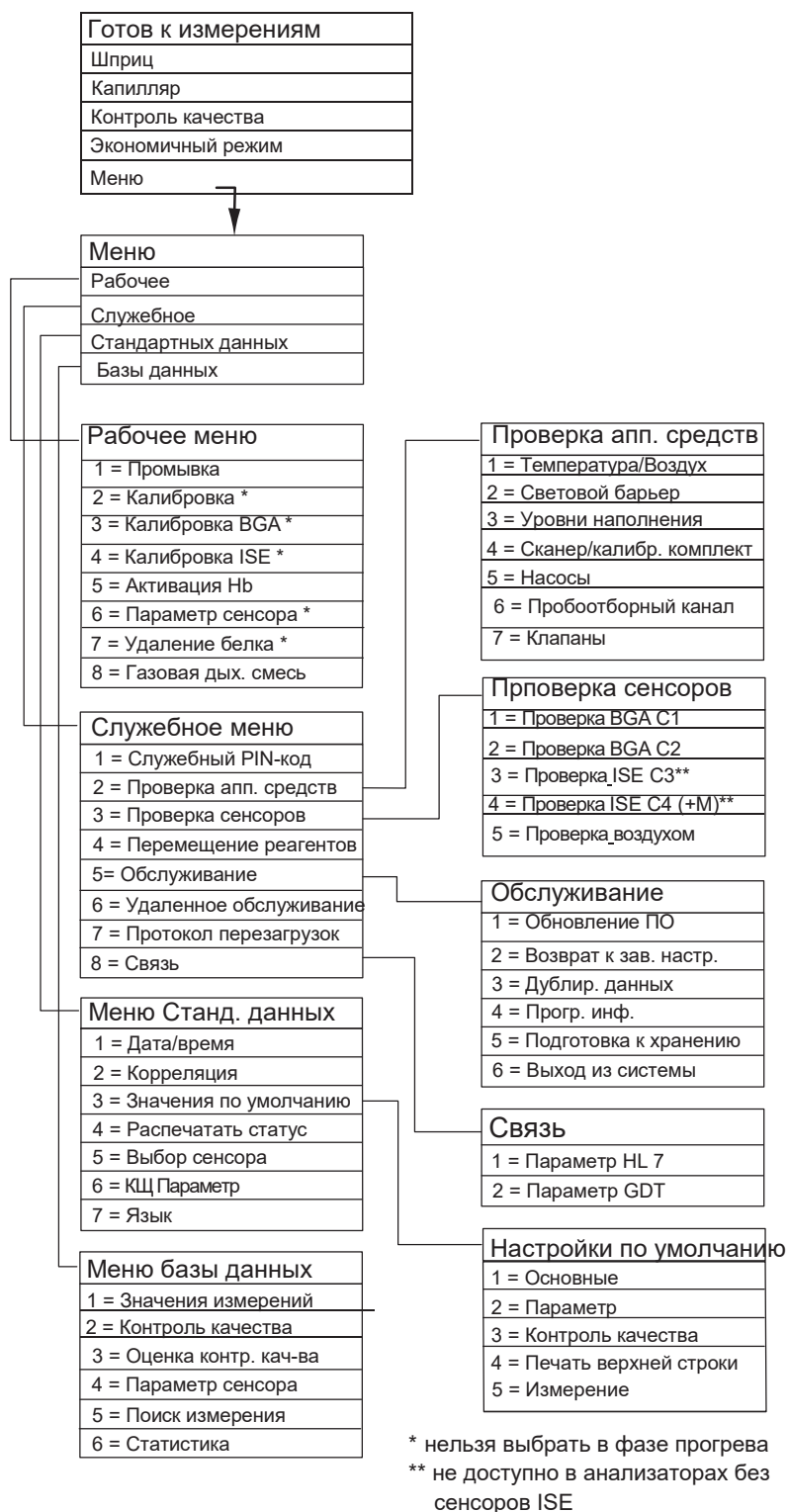
Рисунок 14 Обзор программного обеспечения 3.04.08
