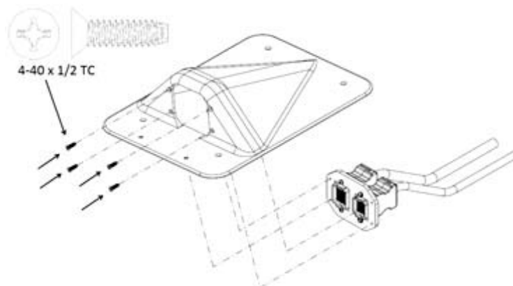
Рисунок 15 — 49. Прикрепление плиты к кронштейну
