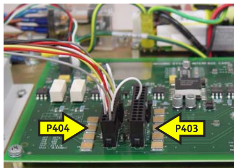
Рисунок 16 - 3. Дополнительный жгут 3016360/60163802 (слева); соединения дополнительного жгута ISI с разъемами P404 и P403 (справа)
