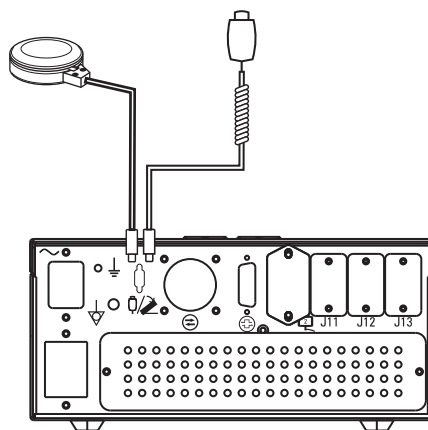
Рисунок 15 — 31. Расположение блока питания с ручным и педальным переключателями
