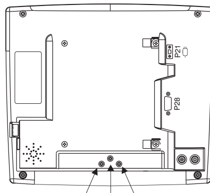
Рисунок 15 — 17. Задняя панель блока управления дисплеем — снимите винты
