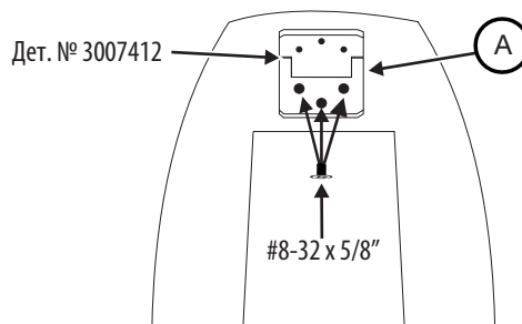
Рисунок 15 — 15. Прикрепите кронштейн (А) к стойке блока управления дисплеем
