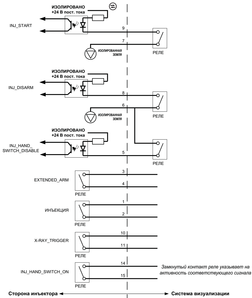
Рисунок 17 — 2. Универсальный кабель ISI
