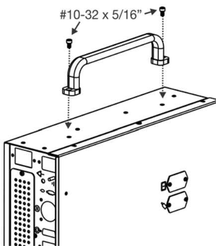
Рисунок 15 — 13. Прикрепите ручку
