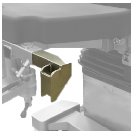
Рисунок 7.1 – Держатель секции ножной 202.040 (версия для ОК-Теты, ОМ-Сигмы)
