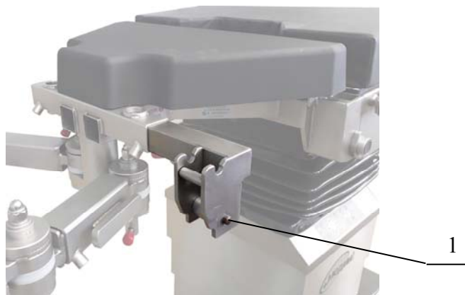
1 – фиксатор (версия для ОК-Теты, ОМ-Сигмы)
