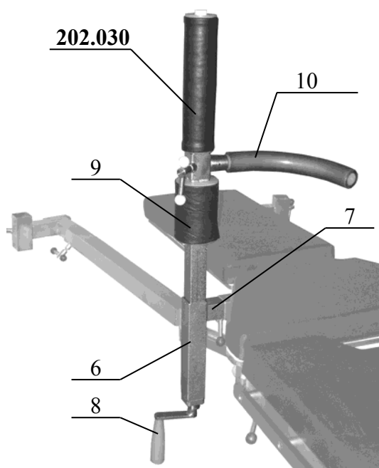
Рисунок 2. Устройство подъема с промежуточной опорой (опорой бедра).
