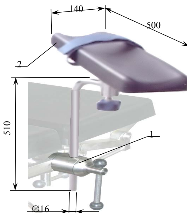
Рисунок 1. Комплект КПП-15 для операций с верхним позиционированием руки.
