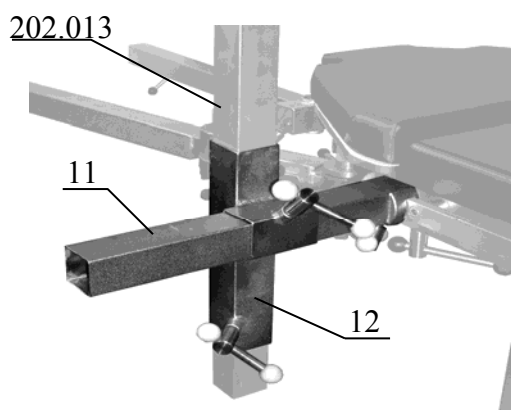
Рисунок 4. Адаптер механизма натяжения для бокового крепления к столу
