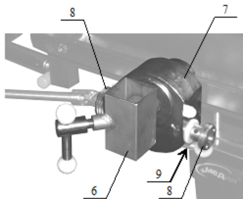
Рисунок 2 - Редуктор с поворотным зажимом штанги подколенной опоры
