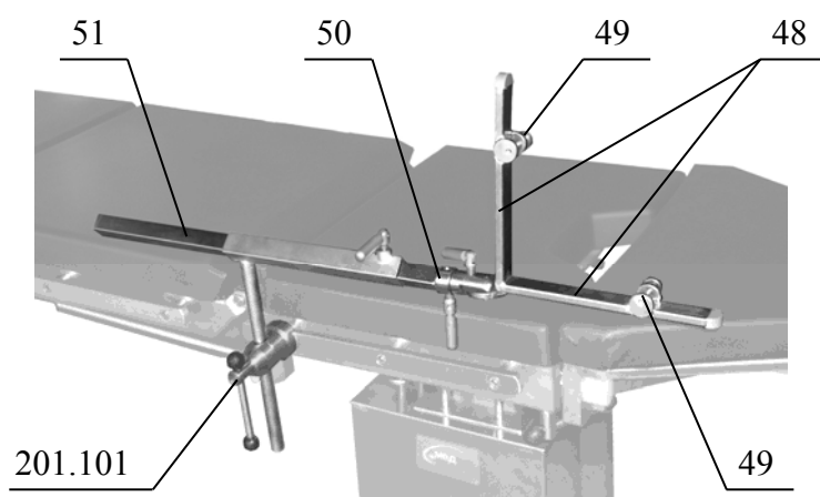
Рисунок 11 – Держатель рентгеновской кассеты 202.041
