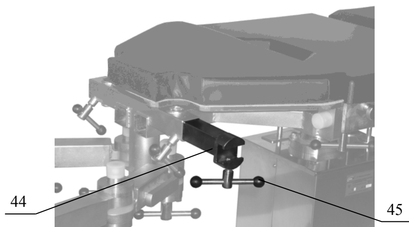
Рисунок 7 – Держатель секции ножной 202.040
