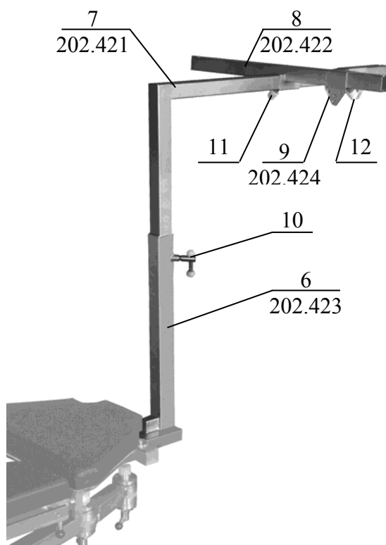
Рисунок 2 - Стойка опорная с перекладиной для подвешивания
