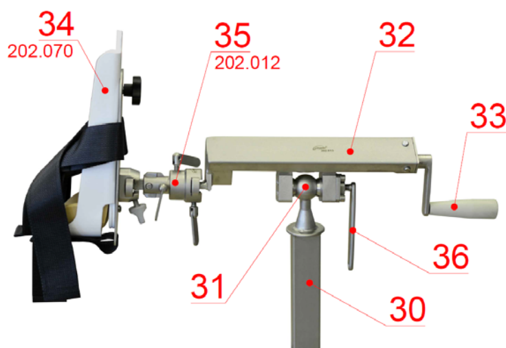
Рисунок 3 – Механизм натяжения
