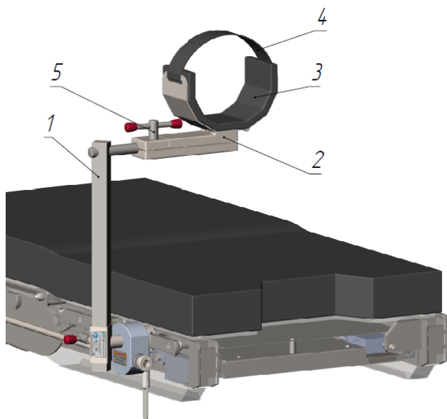
Рисунок 1 - Подколенная опора с регулируемым ложем для бедра
