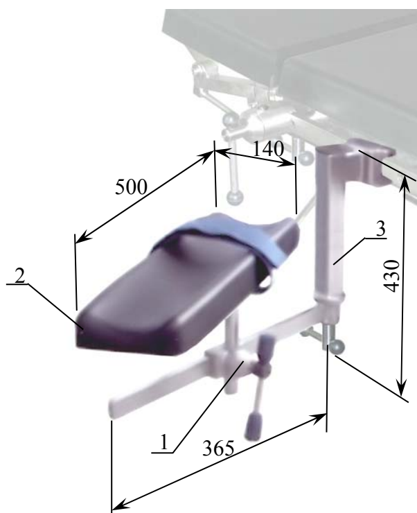
Рисунок 1. Комплект КПП-16 для операций с нижним позиционированием руки.
