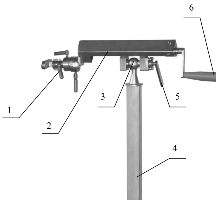
Рисунок 1. Комплект КПП-08 для тракция костей.
