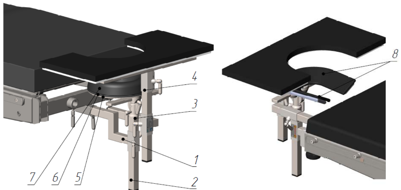
А – Комплект приспособлений
