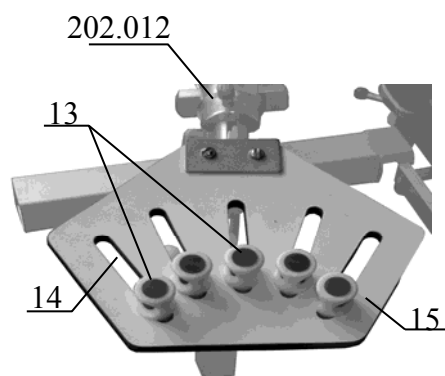
Рисунок 5. Манжета для фиксации кисти (фиксатор Вайнбергера)
