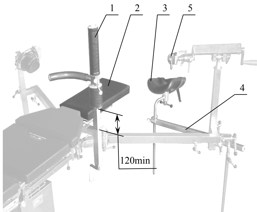
Рисунок 1. Комплект КПП-03 для орто-травматологических операций на бедре (дополнение базового).
