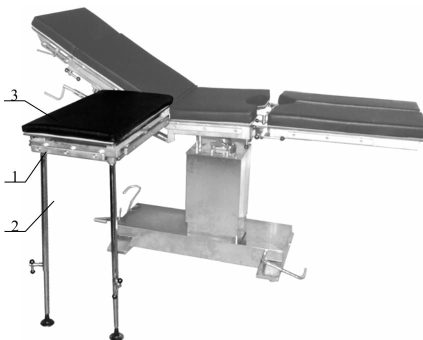
Рисунок 1. Комплект КПП-17 для операций с боковым позиционированием руки.
