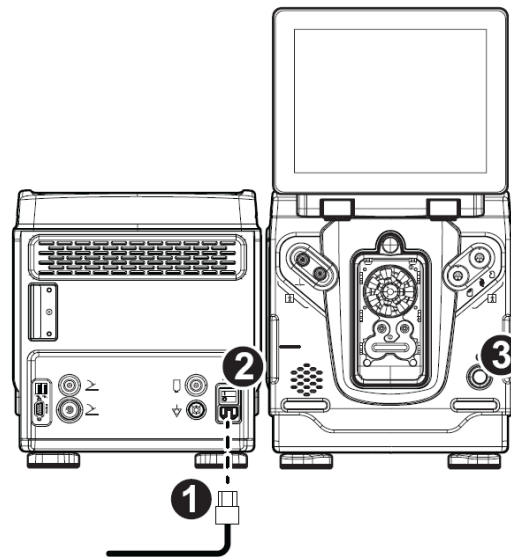
Рисунок 2-5 Подача электропитания
