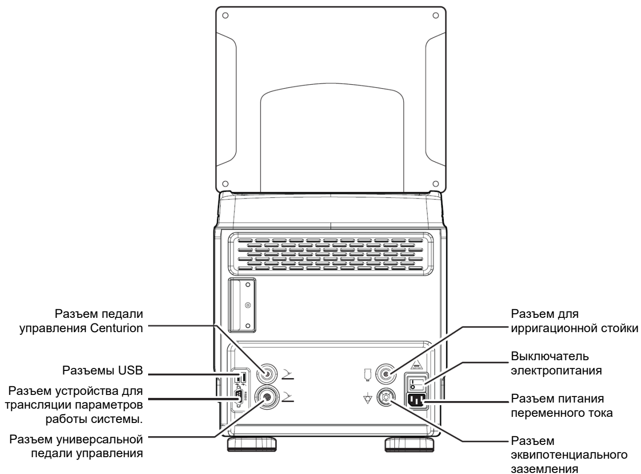
Рисунок 2-3 Задняя панель
