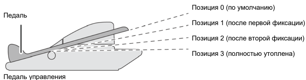
Рисунок 2-8 Позиции педали управления
