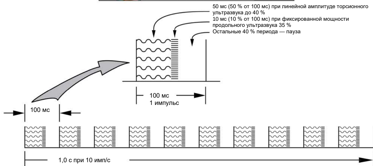
Рисунок 2-74 Экран хирургии импульсной фазоэмульсификации и диаграмма тактирования В данном случае торсионные колебания передаются при 40 % амплитуде в течение 50 мс, продольная мощность передается при 35 % мощности для 10 мс, нет мощности/колебаний передается в течение 40 мс.
