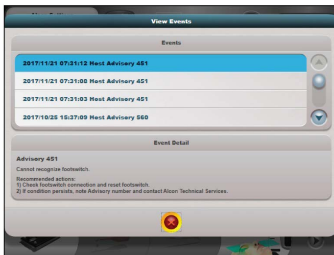
Рисунок 2-58 Диалог просмотра событий
