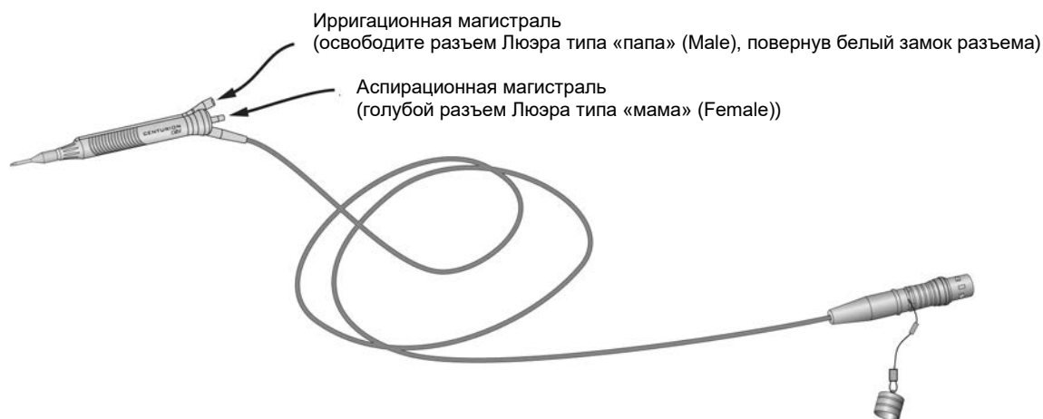
Рисунок 3-3 Подсоединение ультразвуковой рукоятки к тубингу кассеты для факэмульсификации и к панели соединителей системы LEGION (показана рукоятка Centurion OZil).
