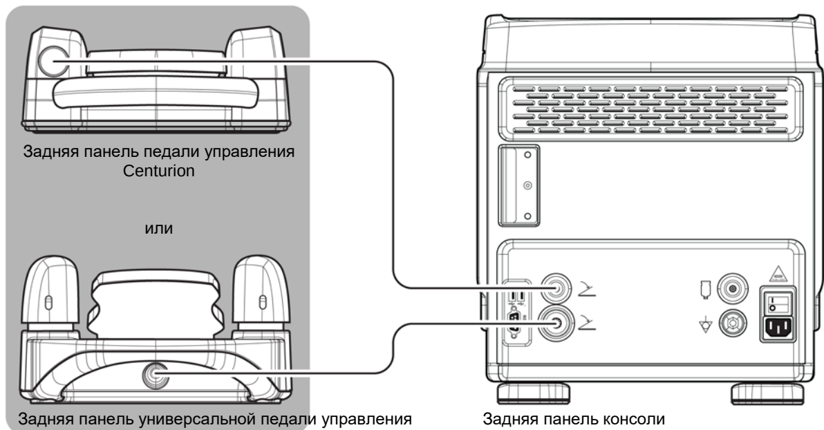
Рисунок 2-7 Разъемы кабеля для педали управления
