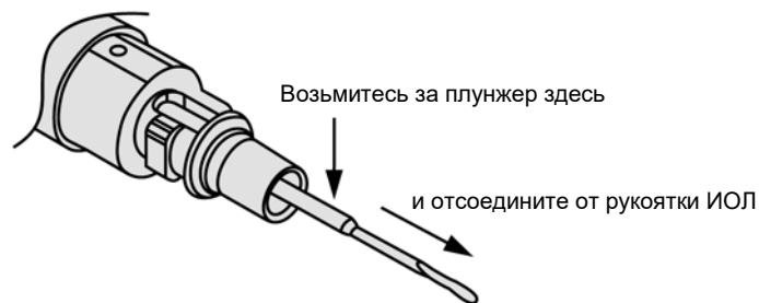
Рисунок 3-7 Удаление плунжера из рукоятки-инжектора ИОЛ Intrepid AutoSert .
