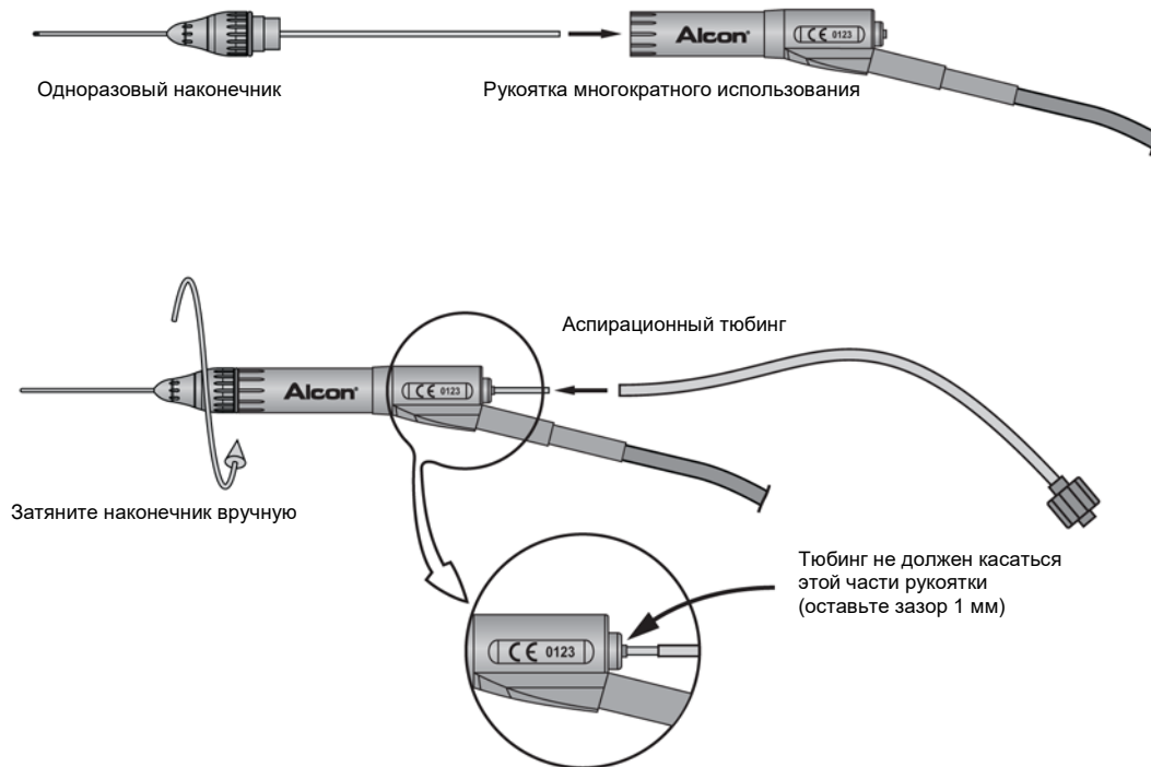
Рисунок 2-18 Рукоятка для витректомии
