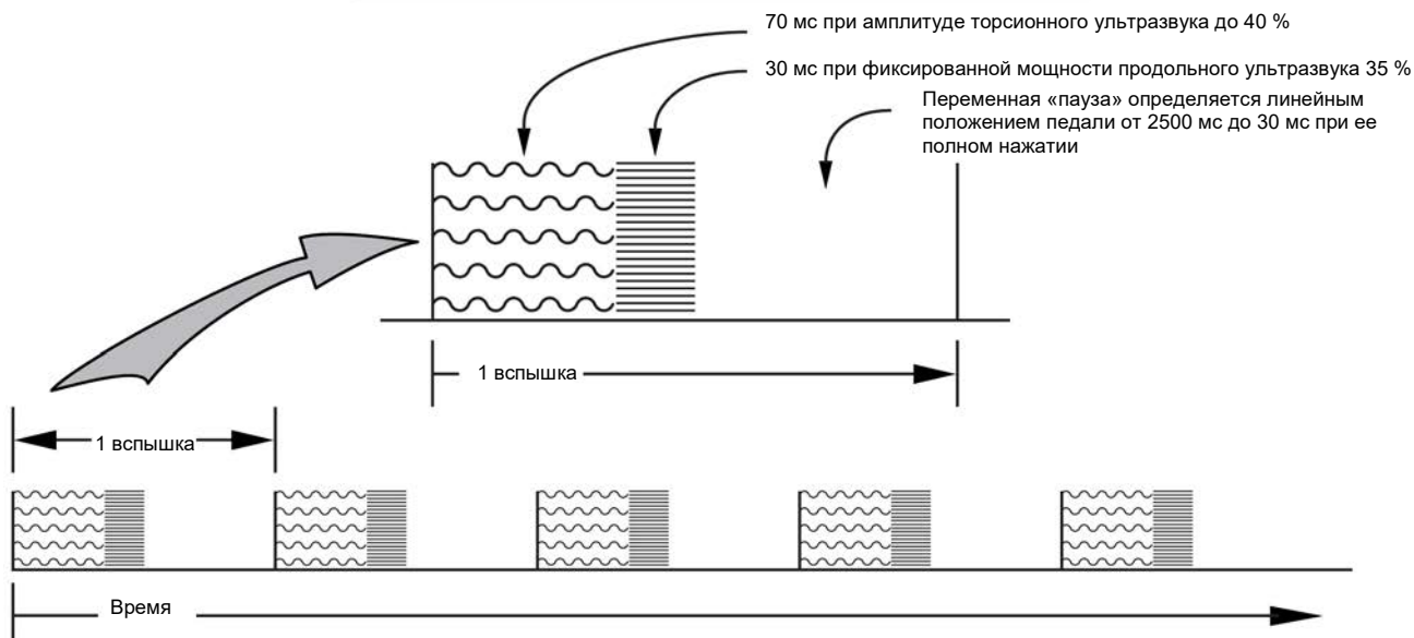
Рисунок 2-75 Экран хирургии факэмульсификации «вспышка» и диаграмма тактирования В данном случае торсионные колебания подаются при 40 % амплитуде на 70 мс, продольная мощность подается при 35 % мощности на 30 мс, а пауза уменьшается по мере нажатия педали в диапазоне хода 3.
