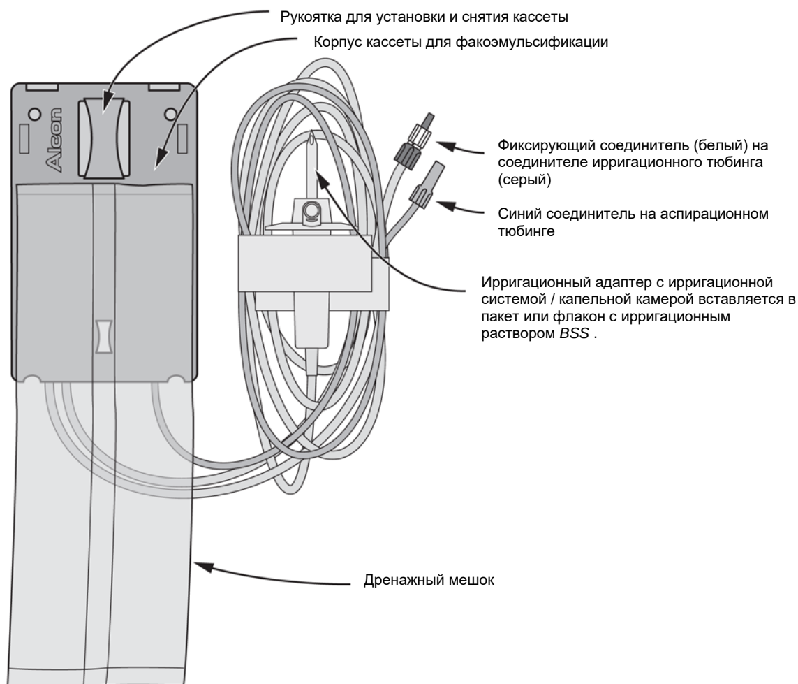
Рисунок 2-19 комплект LEGIONFMS (англ. Fluidics Management System)
