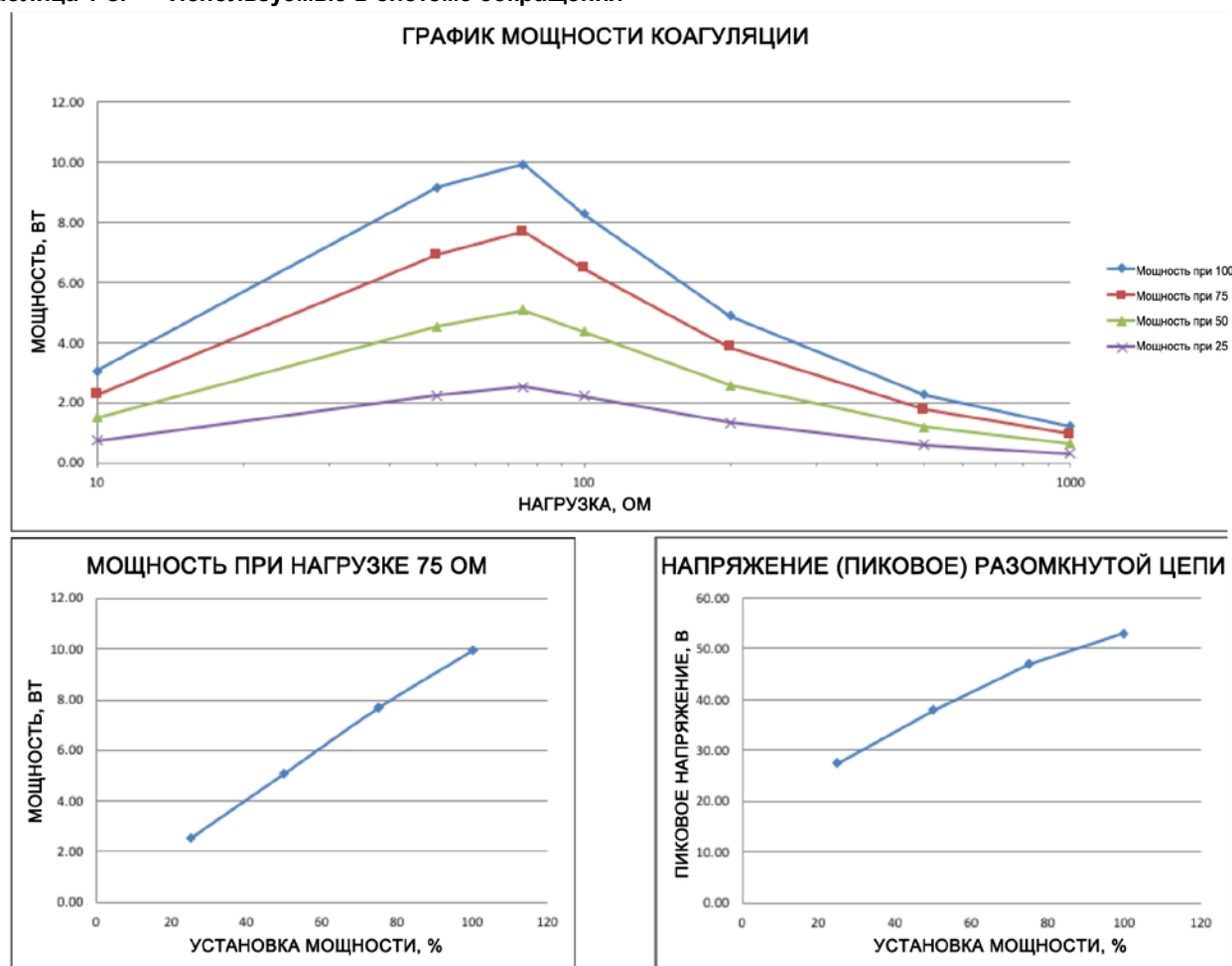
Рисунок 1-4 Выходная мощность коагуляции
