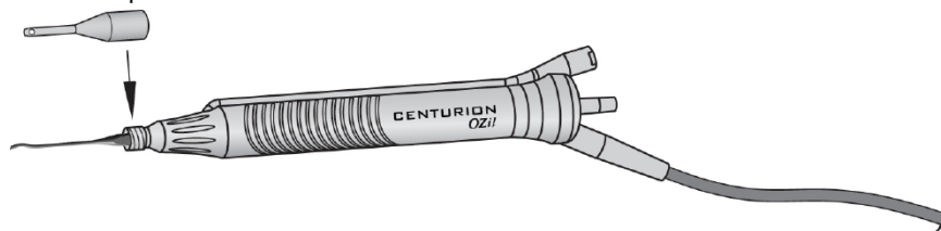
Рисунок 2-14 Рукоятка Centurion OZil с ирригационным сливом
