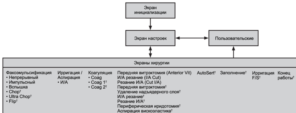
Рисунок 2-24 Навигация в экранах пользователя системы LEGION
