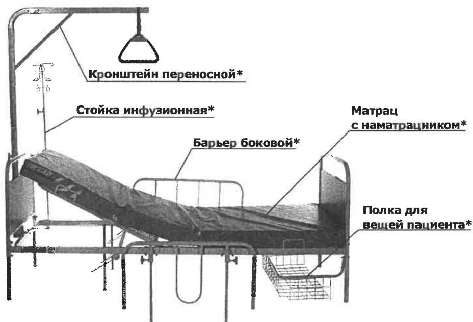
Рисунок 2 – Общий вид кроватей ИЯУБ 25.19-02, ИЯУБ 25.19-03, ИЯУБ 25.19-06, ИЯУБ 25.19-07 в максимальной комплектации (колесные опоры кроватей ИЯУБ 25.19-02, ИЯУБ 25.19-06 условно не показаны)
