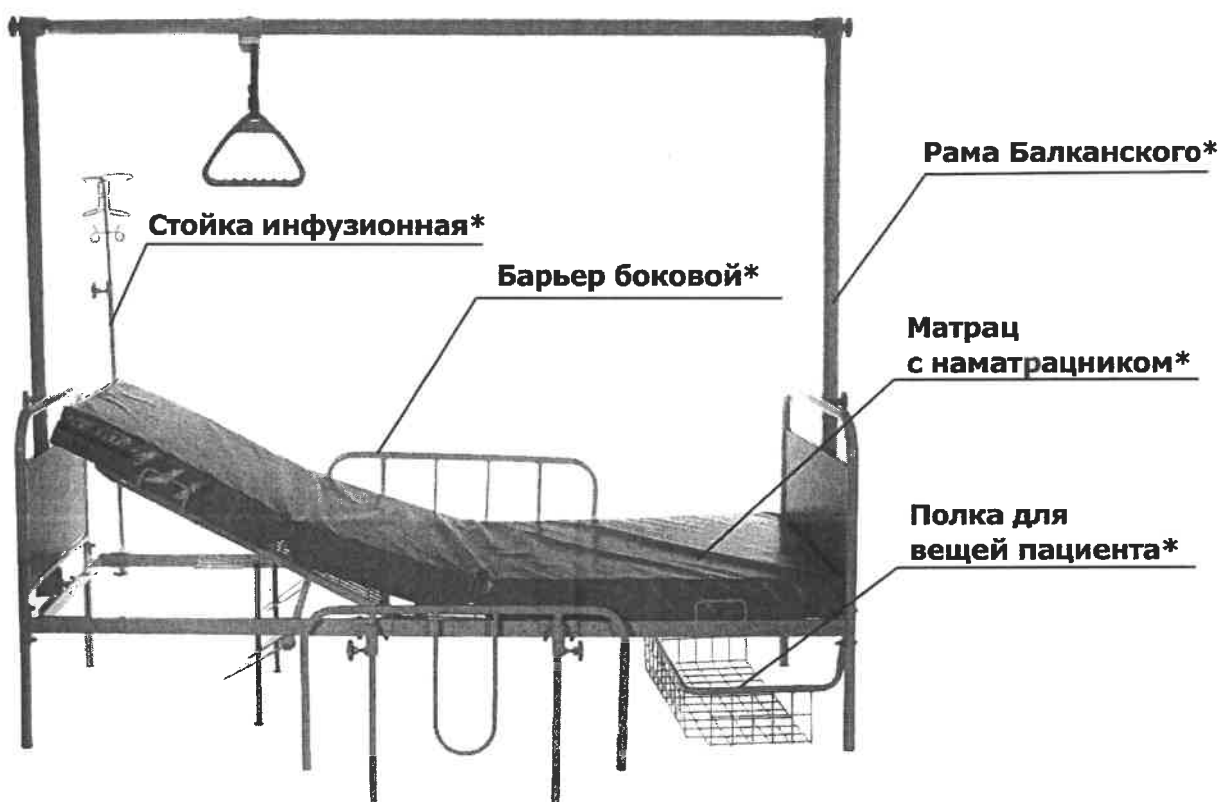
Рисунок 1 – Общий вид кроватей ИЯУБ 25.19, ИЯУБ 25.19-01, ИЯУБ 25.19-04, ИЯУБ 25.19-05 в максимальной комплектации (колесные опоры кроватей ИЯУБ 25.19, ИЯУБ 25.19-04 условно не показаны)
