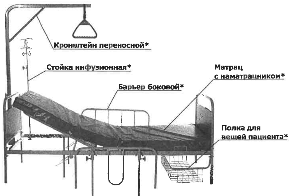
Рисунок 2 – Общий вид кроватей ИЯУБ 21.19-02, ИЯУБ 21.19-03 в максимальной комплектации (колесные опоры кровати ИЯУБ 21.19-02 условно не показаны)
