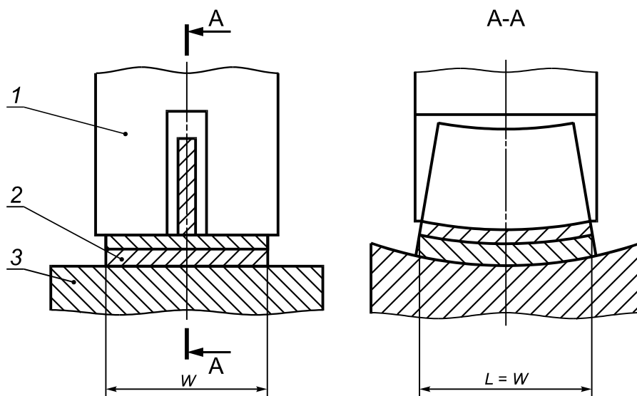
1 — плунжер; 2 — испытуемый образец; 3 — нагревательная плита
