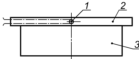
Рисунок 4 — Расположение термодпары при измерении теплопередачи
