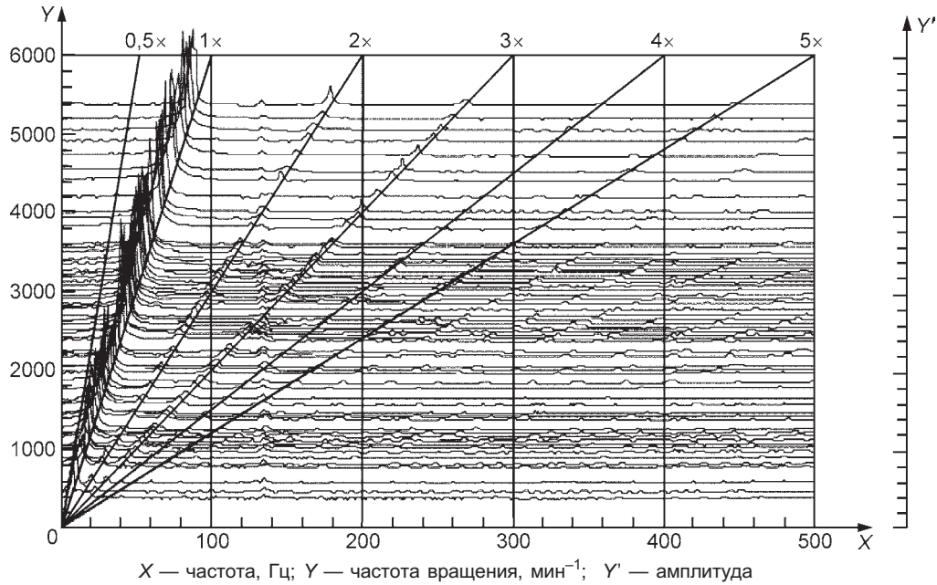
Рисунок 23 — Каскадный спектр
