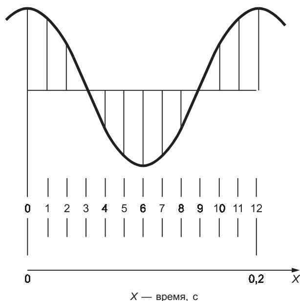
Рисунок 6 — Временная форма сигнала
