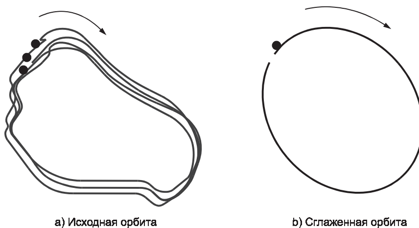
Рисунок 11 — Орбита прецессии вала
