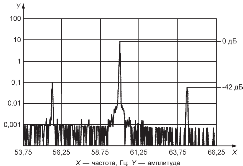
Рисунок 18 — Спектр вибрации неисправного электродвигателя
