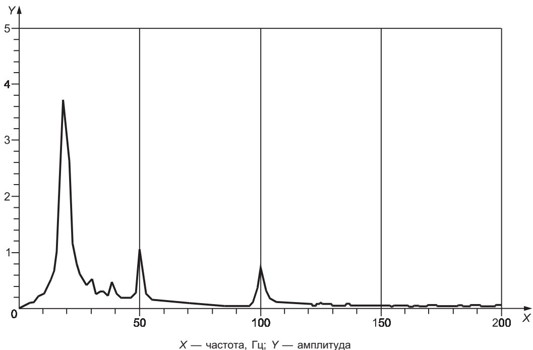
Рисунок 16 — Амплитудный спектр
