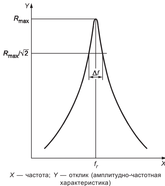
Рисунок 15 — Определение добротности Q
