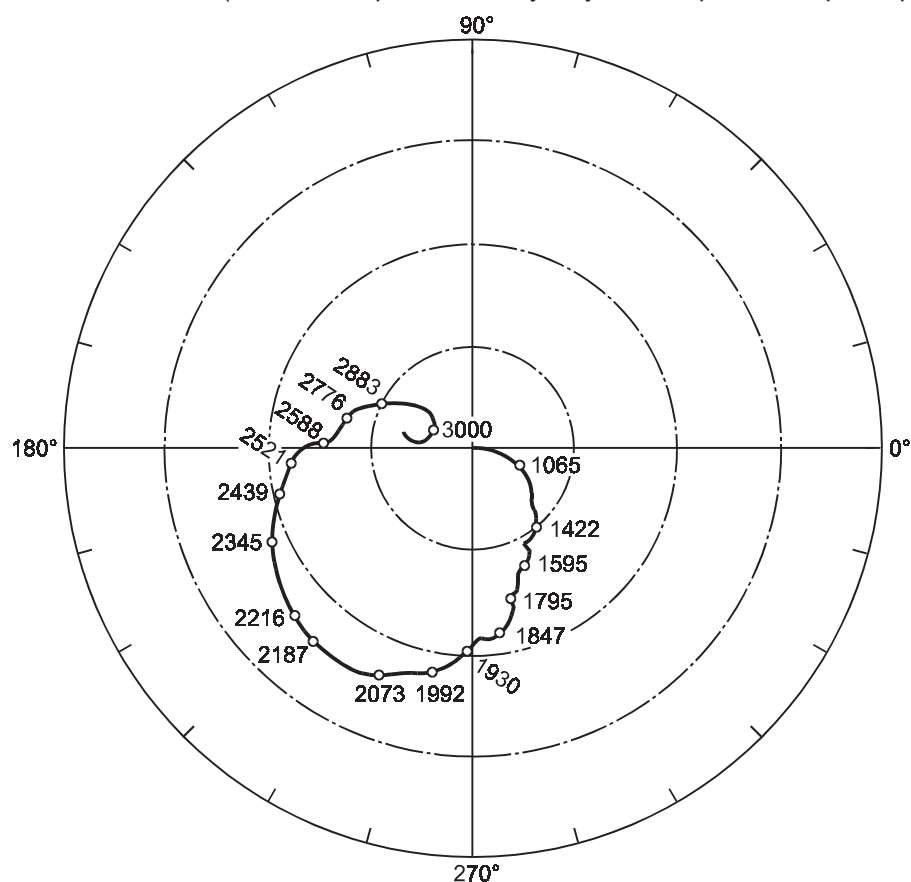
Рисунок 22 — Диаграмма Найквиста
