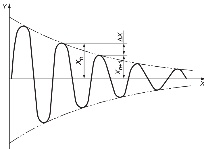
Рисунок 14 — Затухание сигнала вследствие демпфирования в системе
