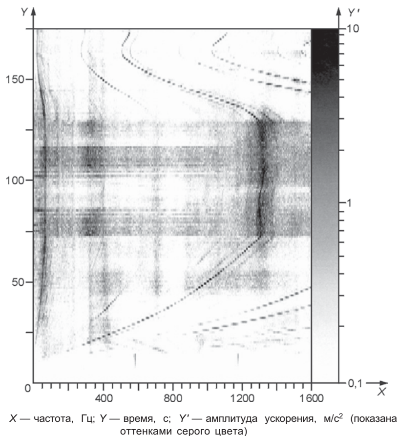
Рисунок 25 — Двумерная спектрограмма
