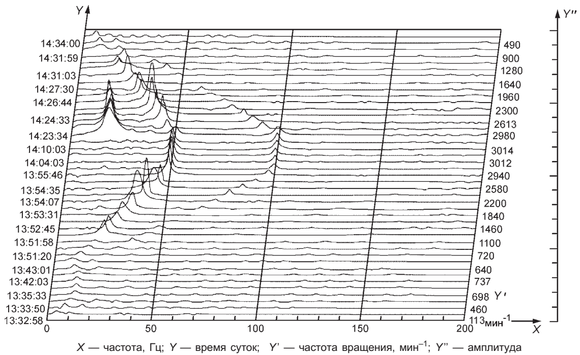
Рисунок 24 — Каскадный спектр вибрации турбины
