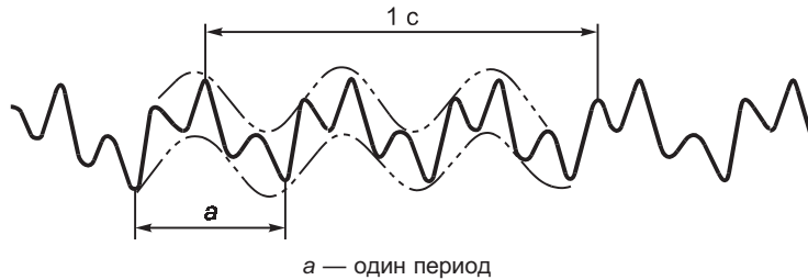
Рисунок 7 — Суперпозиция сигналов
