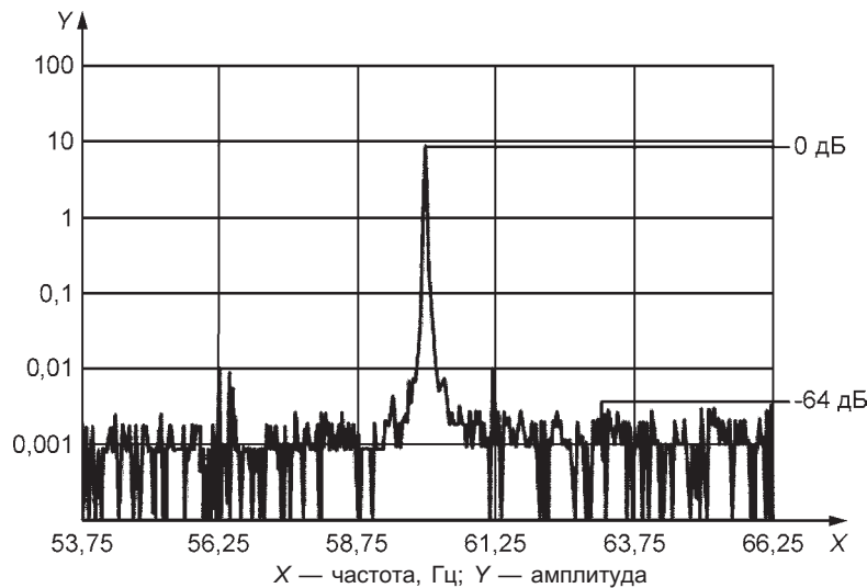
Рисунок 17 — Спектр вибрации исправного электродвигателя
